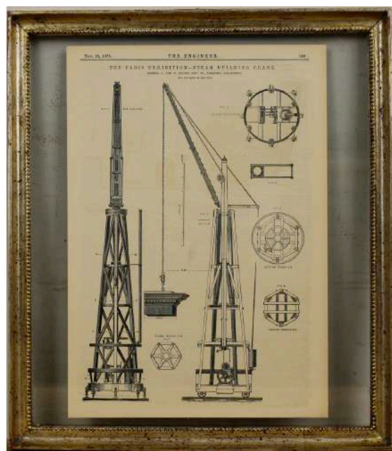
228 | Gru da cantiere della Fonderia Oreteia Scheda descrittiva pubblicata sulla rivista “The Engineer” del 22 novembre 1878, pag. 369. Prezzo base d’asta 100,00 €
